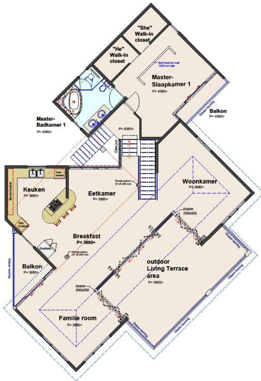
Plattegrond 1ste Verdieping
